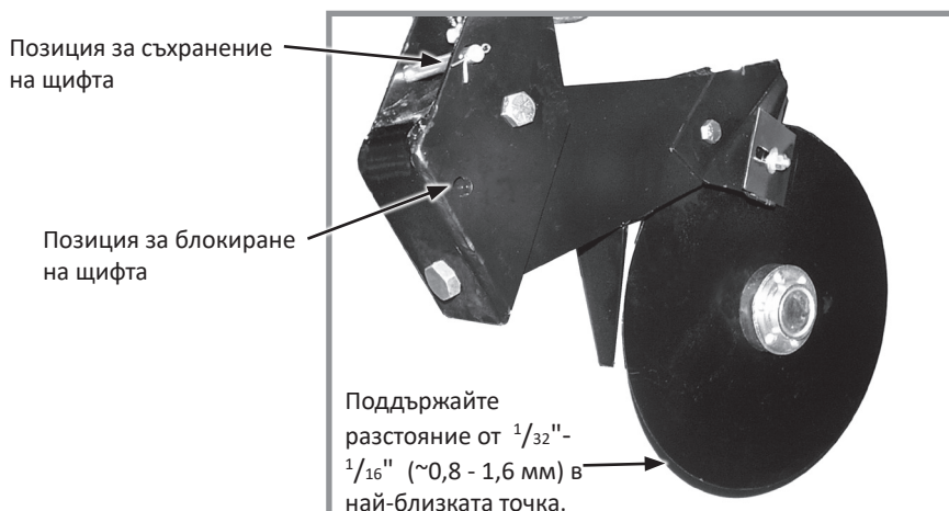
Лемеж за тор с два диска
