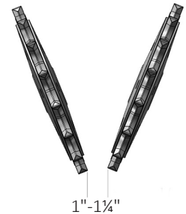
Монтирана на сеещата секция натискателната ролка с шипове
