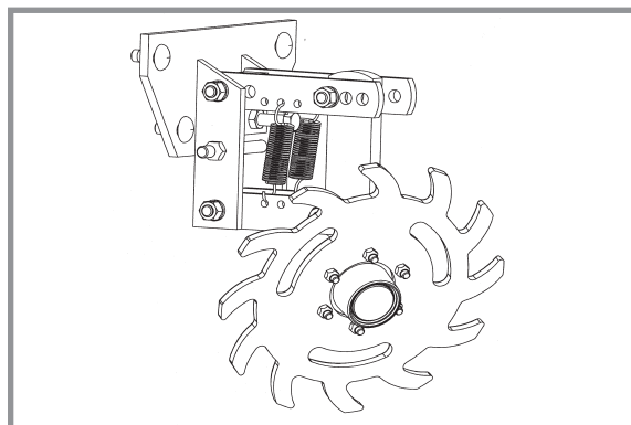
Монтирани на сееща секция колела за сътрещица
