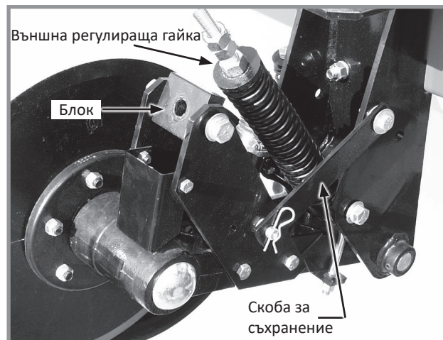
Фиксиране на подсилен едnodисков лемеж
