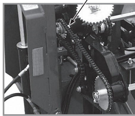
Задвижваща система за сух тор
