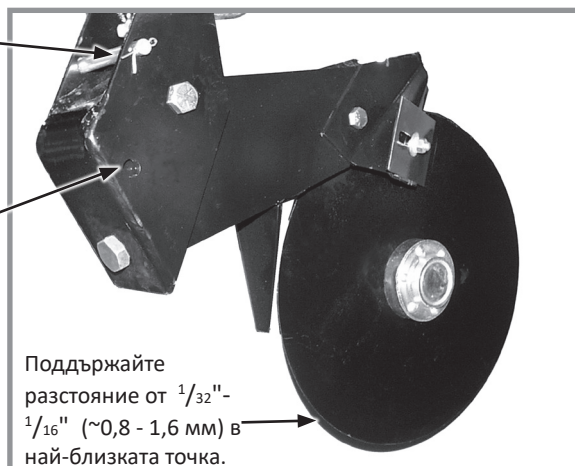
Лемеж за тор с два диска
