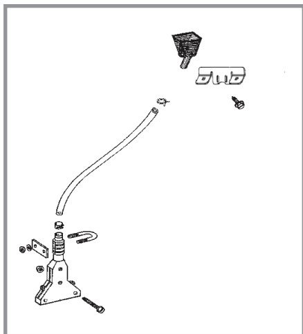
Приставка за 4 1/2" (~12 см) ленточна обработка с компенсиране на наклона
