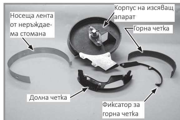
Частите на изсяващ апарат тип четка
