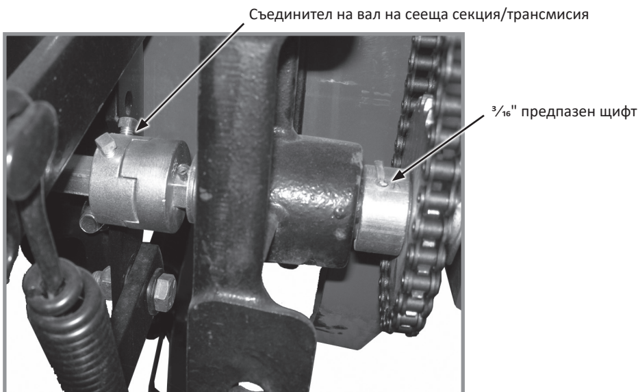
Соединител на вал на трансмисия и вал на сееща секция
