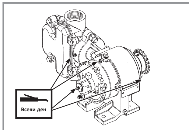
Бутална помпа за течен тор - 4 (пълнете външния салник, докато смазочният материал изтече от отвора за източване на дъното.)
