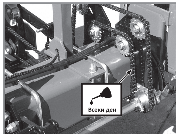
Задвижваща верига на система Interplant (с единична рама)
