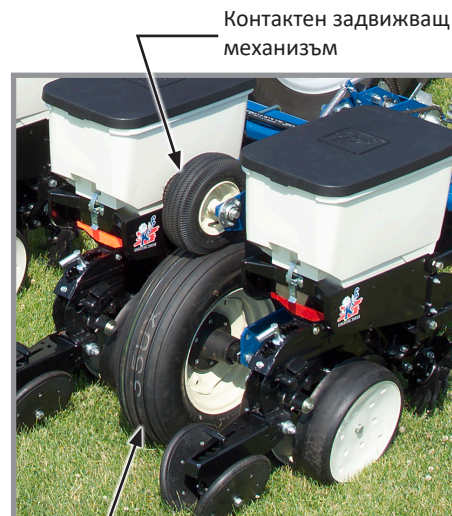
Задвижващ механизъм за транспортиране/полева работа
