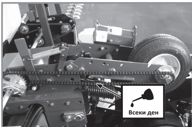
Задвижващи вериги на контактен задвижващ механизъм
