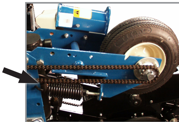
Местоположение на затягащата пружина
