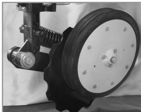
Опорно/габаритно колело на назъбен едnodисков лемеж
