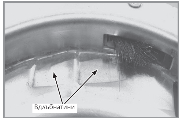
Износена носеща пластина
