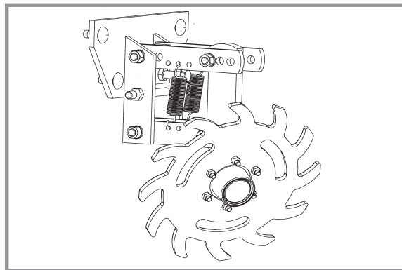
Монтирани на сеещата секция колела за сътренища
