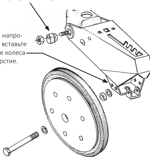
Эксцентриковая втулка
