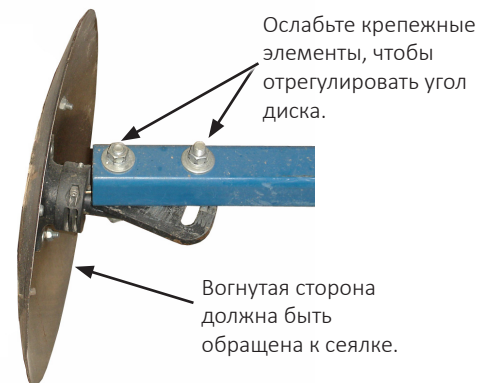
Регулировка угла дискового ножа маркера
