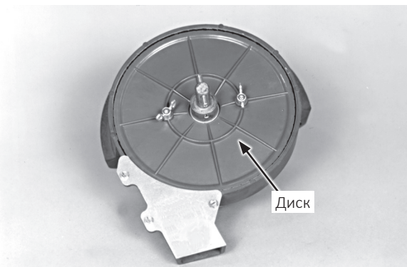
Установленный высевающий диск щеточного высевающего аппарата
