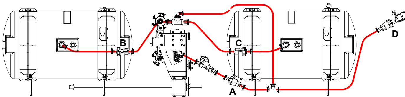
Прокладка трубопроводов оборудования для внесения жидких удобрений
