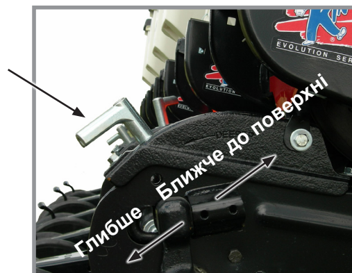
Регулювання глибини висіву
