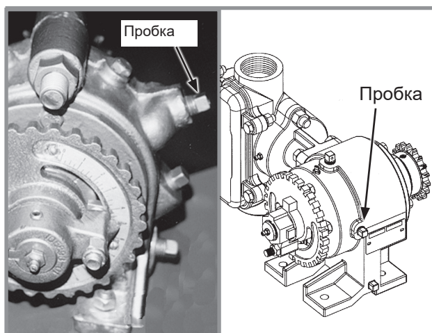
Розташування заливної пробки поршневого насоса
