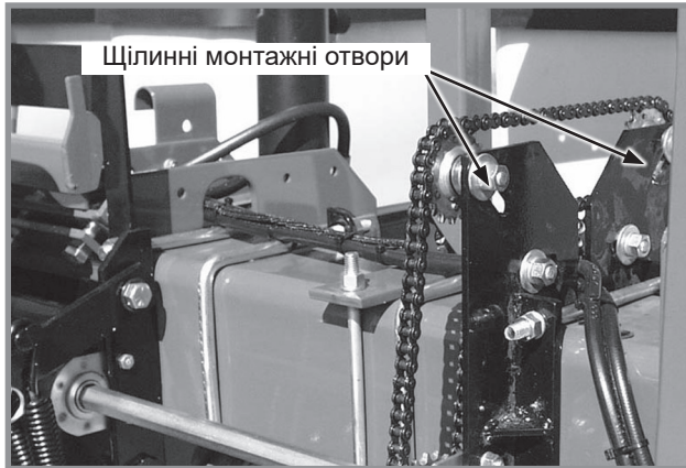
Регулювання натягу ланцюга приводу роздільного висіву
