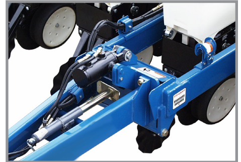
Подовження зчпного пристрою з автоматичним вирівнюванням для роздільного висіву
