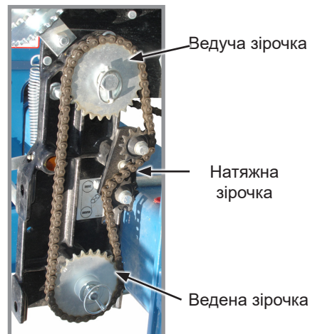
Натяг ланцюга приводу трансмiсії норми висiву
