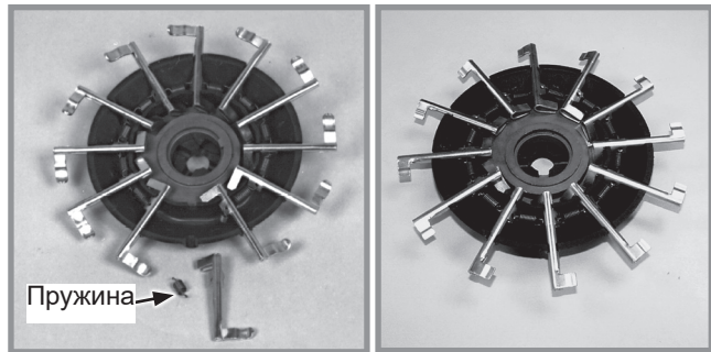
Пальчиковий висівний апарат для кукурудзи (Розташуйте отвір пружини з боку тримача) Пальчиковий висівний апарат для соняшнику олійного зборі
