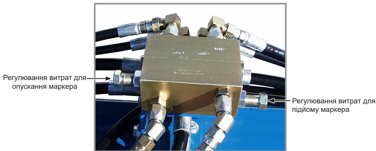
Клапан регулювання витрати маркерів
