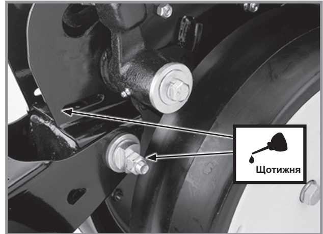
Ексцентрикові втулки (по 2 точки змащення на ряд) V-подібного зашпаровуючого колеса, зашпаровуючих дисків/одиначного прикочуючого колеса і/або причіпного зашпаровуючого колеса висівної секції
