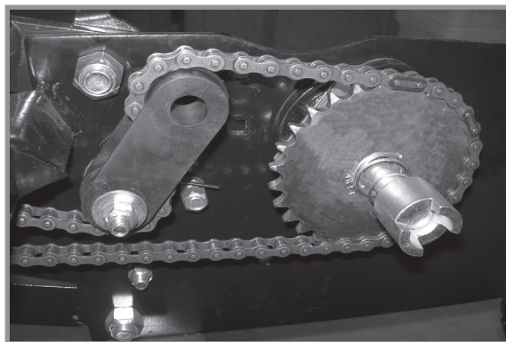
Привід вакуумного висівного апарату фронтальної висівної секції
