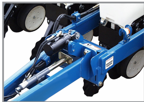
Подовження зчіпного пристрою з автоматичним вирівнюванням для роздільного висіву
