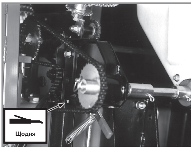
Трансмісія для подачі сухих добрив - по 1 точці змащування на трансмісію
