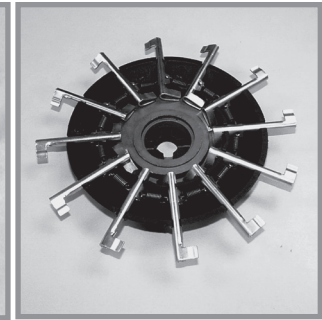
Пальчиковий висівний апарат для соняшнику олійногов зборі
