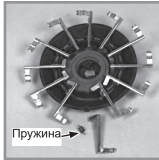
Пальчиковий висівний апарат для кукурудзи (Розташуйте отвір пружини з боку тримача)
