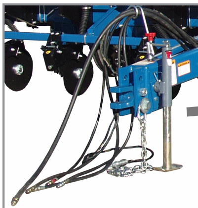
Встановлена підйомна опора
