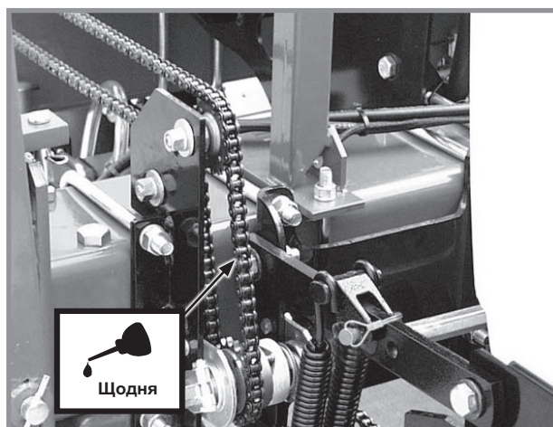
Ланцюг приводу роздільного висіву (подвійна рама)
