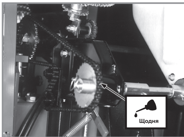
Ланцюги приводу системи внесення сухих добрив
