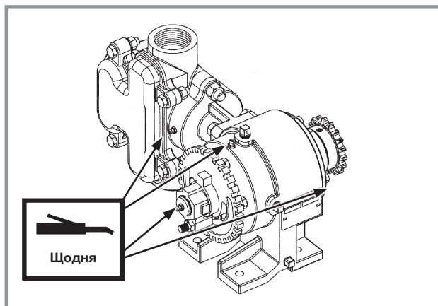
Поршневий насос для рідких добрив - 4 точки змащування (Заповнювати на зовнішньому сальниковому ущільненні, поки мастило не почне витікати через нижній зливний отвір.)
