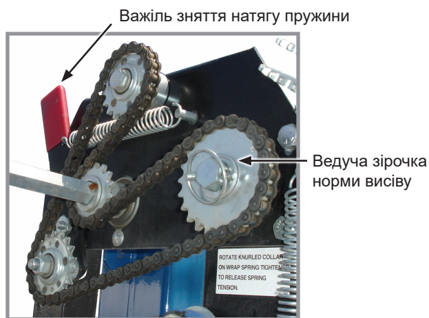
Трансмсія
