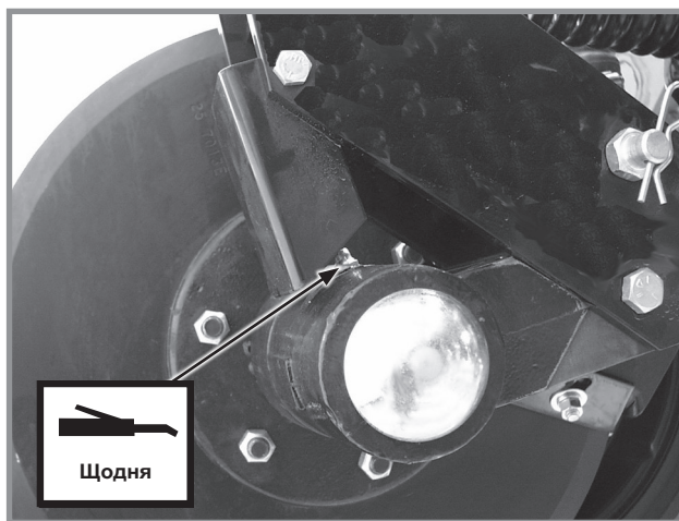
Посилений однодисковий сошник для внесення добрив - 1 точки змащування (Розташований на маточині осі дискового сошника)
