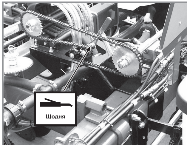
Натяжна зірочка ланцюга приводу поршневого насоса - 1 точка змащування
