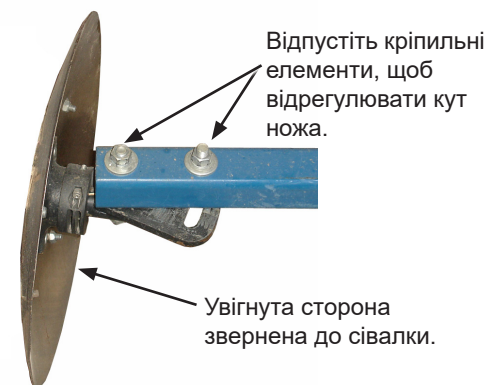
Регулювання кута дискового ножа маркера
