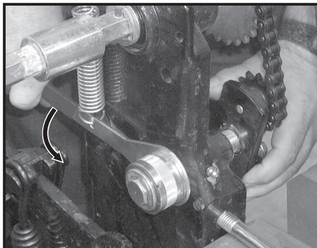
Збільшення натягу ланцюга
