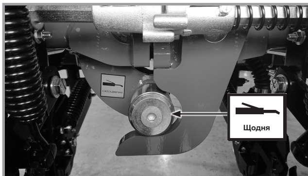
5. Складна рама - по 1 точці змащування на сторону.
