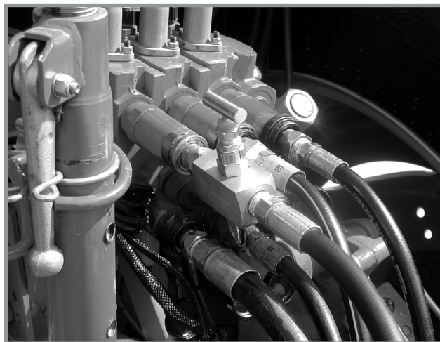
Комплект голчастого клапана G1K426
