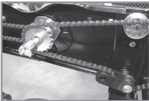
Привід механічного висівного апарату задньої висівної секції
