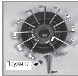
Пальчиковий висівний апарат для кукурудзи в зборі (Положення порожнини пружини відносно держателя)
