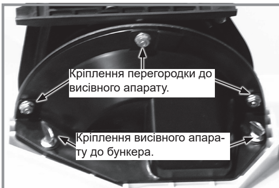
Зняття висівного апарату та перегородки
