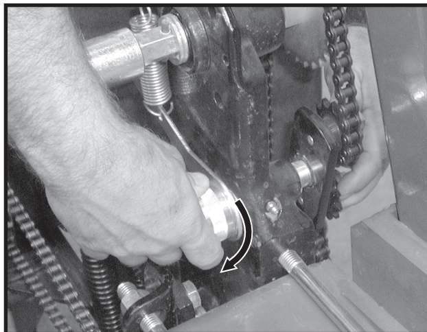
Зняття натягу ланцюга
