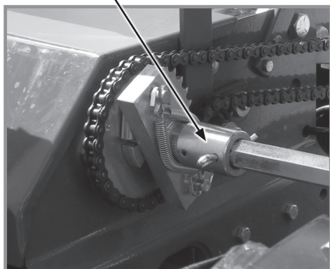
Привід системи внесення рідких добрив
