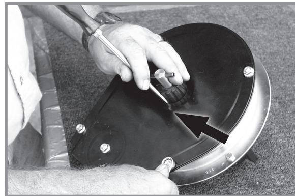
Центрування кришки корпусу стрічки
