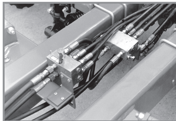
Клапан перемикач
