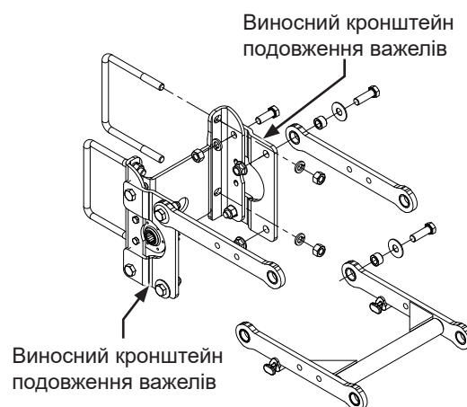
Виносні кронштейни подовження важелів висівних секцій
