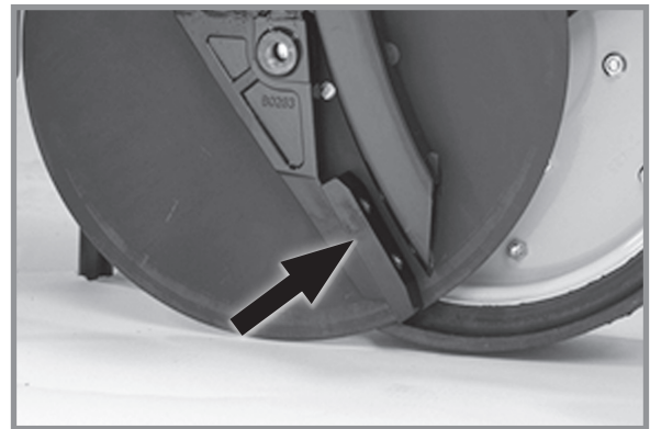
Захист насіннєпроводу/внутрішній чистик (Копіююче колесо/дисковий ніж сошника для внесення насіння знятий)
