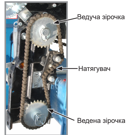
Натяг ланцюга приводу трансмісії норми висіву
