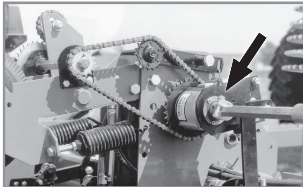
Муфта відключення вказівного ряду
