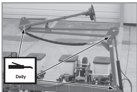
1. Вузли маркерів - по 3 на вузол
