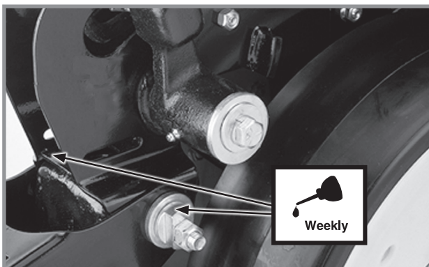
Ексцентриккові втулки (по 2 точки змащування на ряд) V-подібного зашпаровуючого колеса і/або причіпного зашпаровуючого колеса висівної секції
