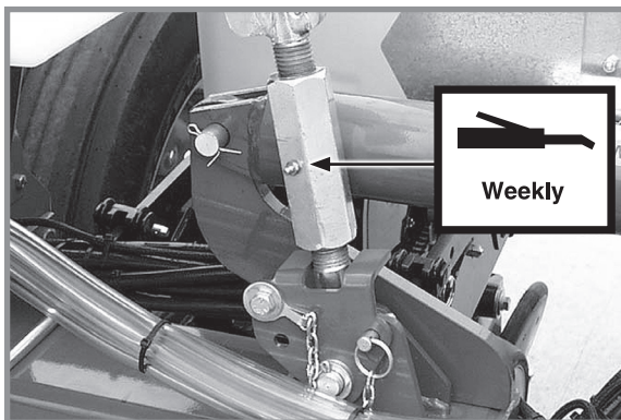
6. Стяжна муфта 1
