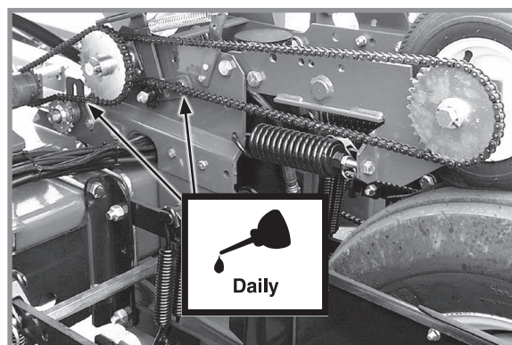
Ланцюги приводу поршневого насоса для рідких добрив
