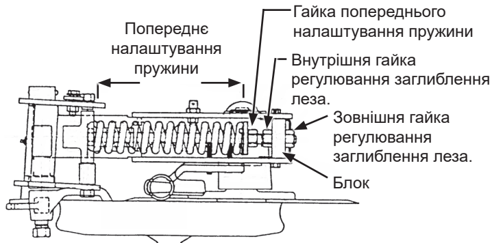
Показано правосторонню конфігурацію (вид зверху)
