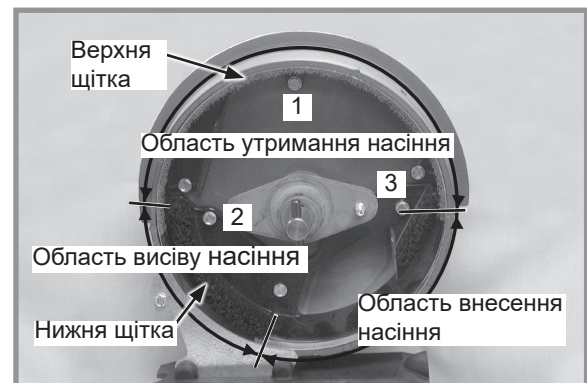
Встановлення фіксатора верхньої щітки
