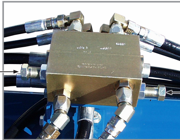
Клапан регулювання витрати маркерів
