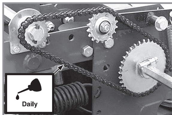
Ланцюги (реверсивні) первинного валу
