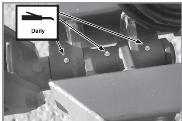
5. Гнучкий штифт дишла - 3
