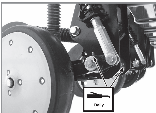
Посилений одnodисковий сошник для внесення добрив - 2 (Розташовані на важелі колеса та кріпленні сошника)
