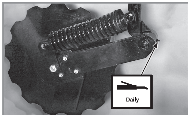
Зубчастий одnodисковий сошник для внесення добрив - 1
