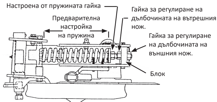
Показана е конфигурацията отъдно (изглед отгоре)
