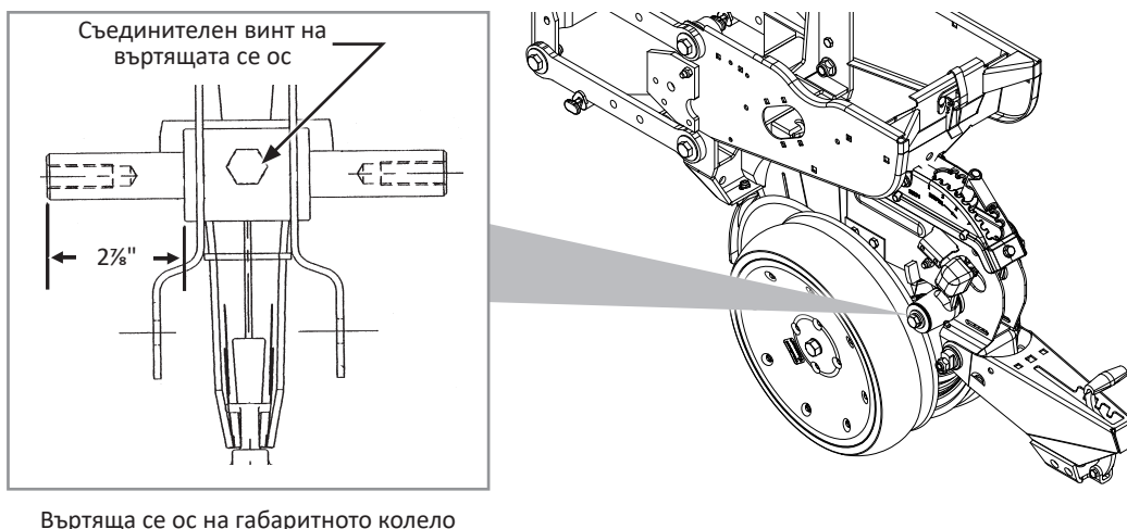
Въртяща се ос на габаритното колело
