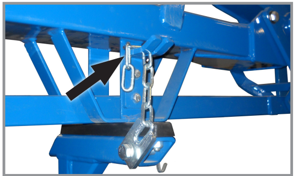
Блокиращо устройство на маркер
