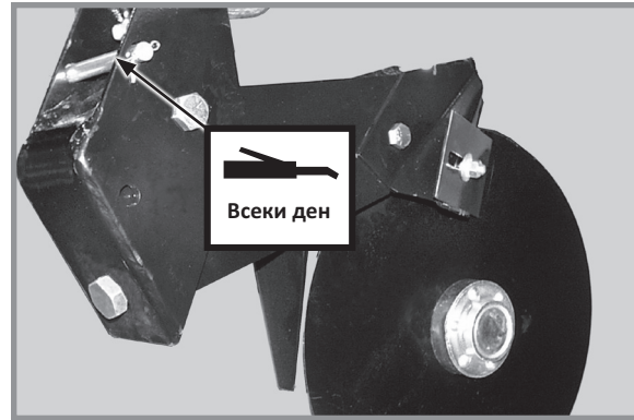
Лемеж за тор с два диска - 1
