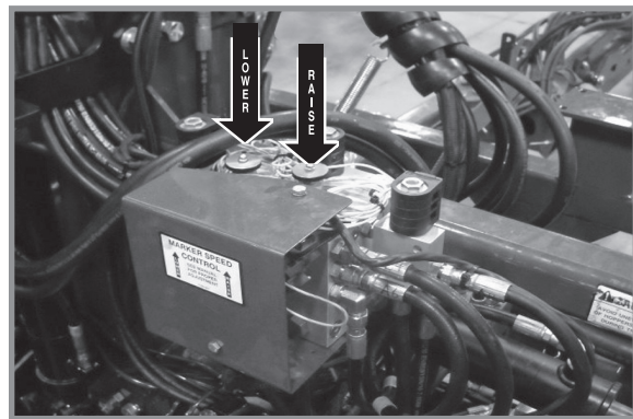
Регулиране на контрола на скоростта на маркерите
