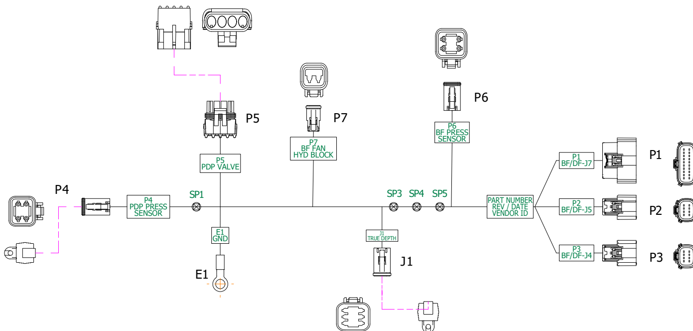
Схема за свързване на проводници, P/N 10260101
