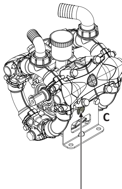
Отстранете пробката, за да източите маслото
