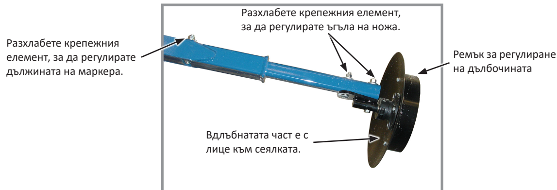
Регулиране на ъгъла на дисковия нож на маркера
