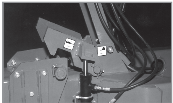
Блокиращ механизъм на теглич
