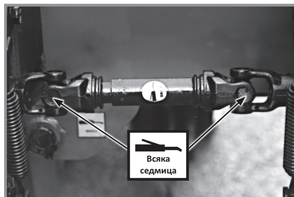
Карданни съединения - 2 на панта
