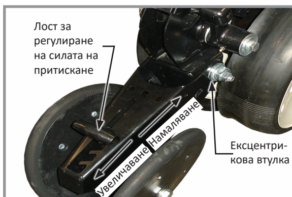
Регулиране на V-образните натискателни ролки
