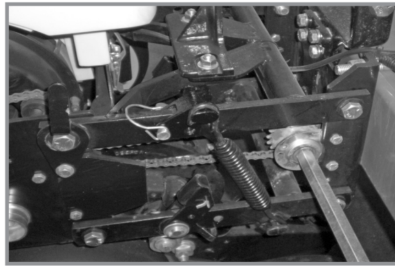
Помощни пружини на фронтална сееща секция
