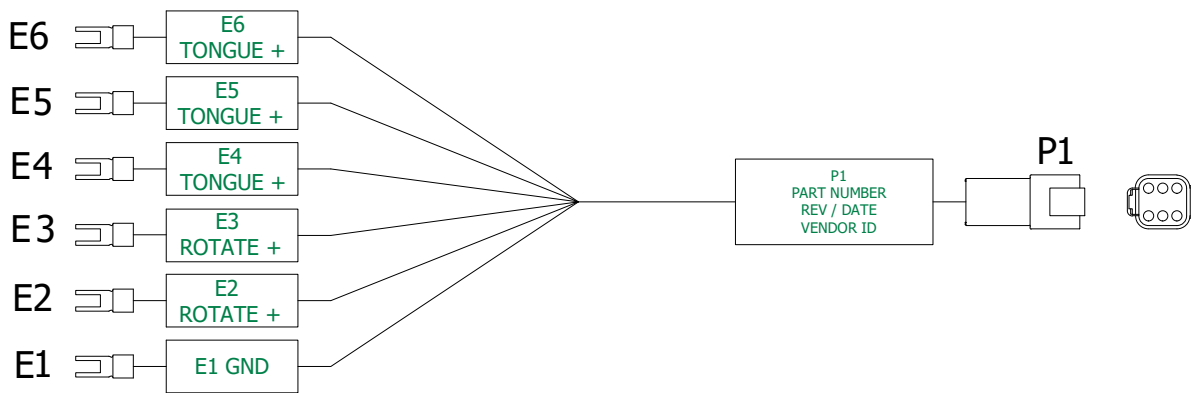
Схема за свързване на проводници, P/N 10150201
