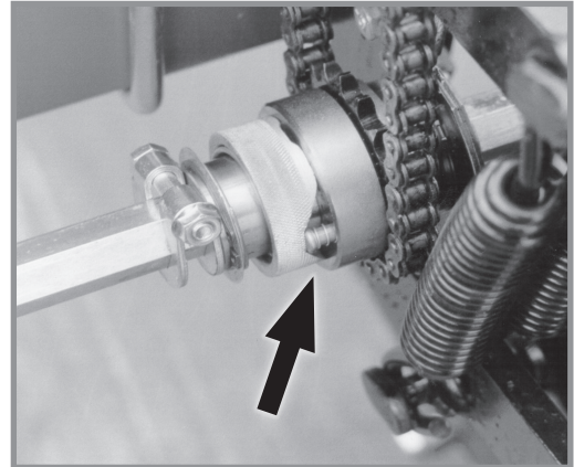
Верижно зъбно колело на система за разделяне на редовете
