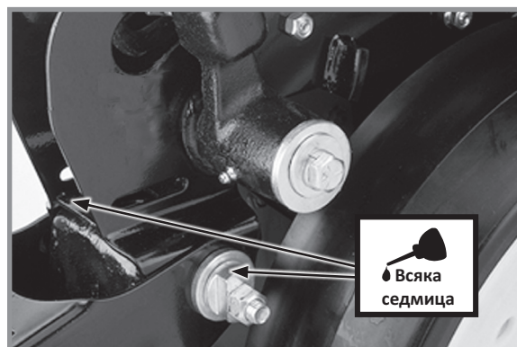
V-образно затварящо колело на сееща секция и/ или ексцентрикови втулки на затварящо колело за зариване на бразди (2 точки на смазване на сееща секция)
