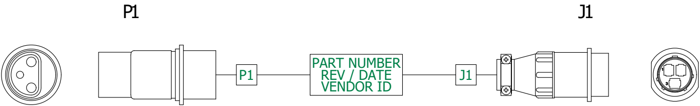
Схема за свързване на проводници, P/N A26751
