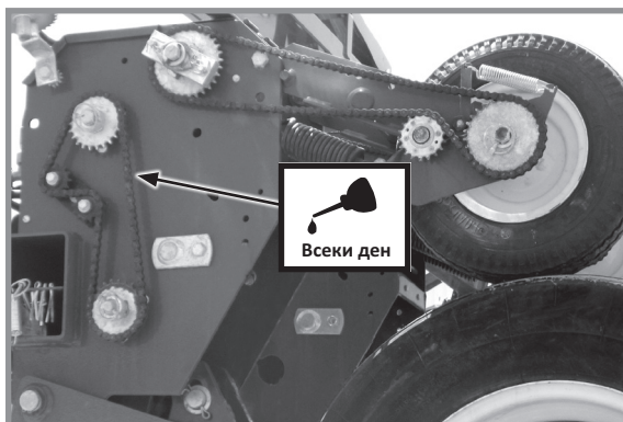
Задвижващи вериги на контактен задвижващ механизъм
