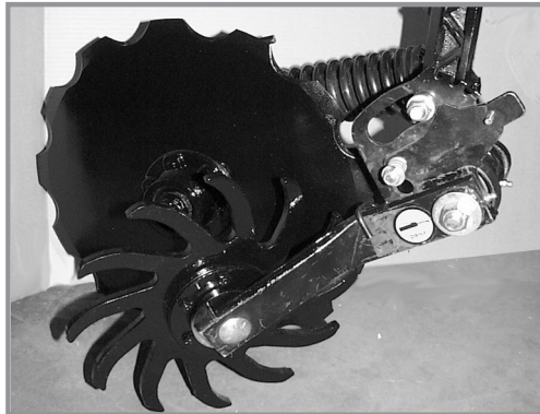
Приставка на колело за сърнища на назъбен еднодисков лемеж
