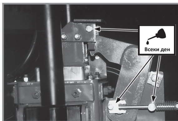
Предпазен щифт в горната част на центъра
