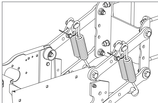
Четири пружини на ред (четворни) (само за монтирани за сеещата секция предпужници с нулева обработка)
