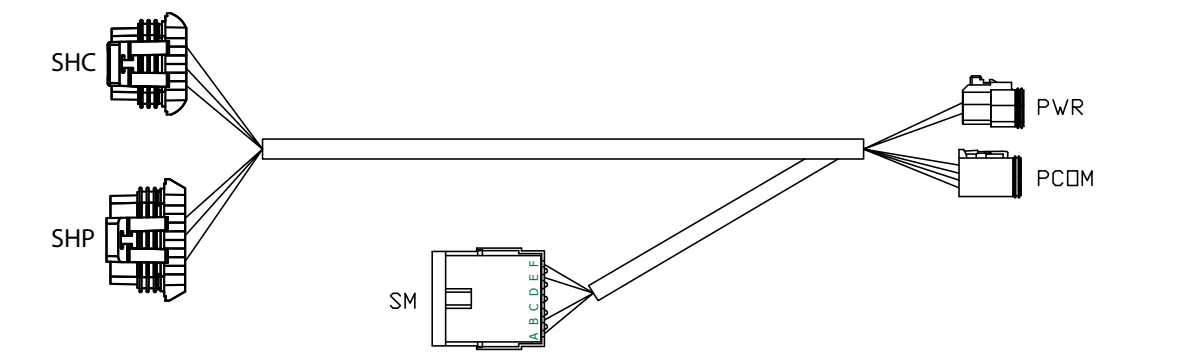
Схема за свързване на проводници, P/N A19388
