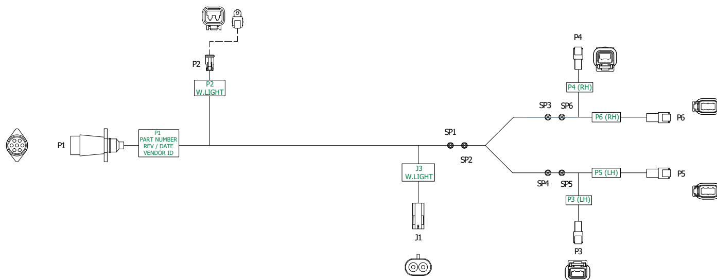
Схема за свързване на проводници, P/N 10174301
