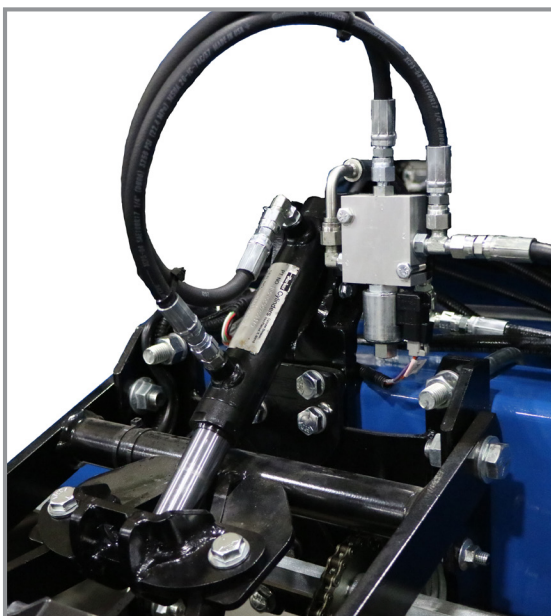
Цилиндър True Depth
