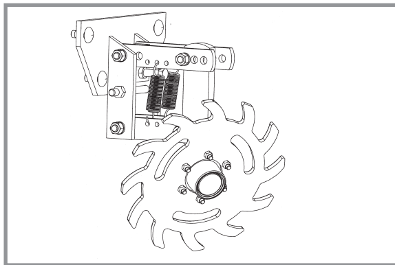
Монтирано на сеещата секция кола за сърнища
