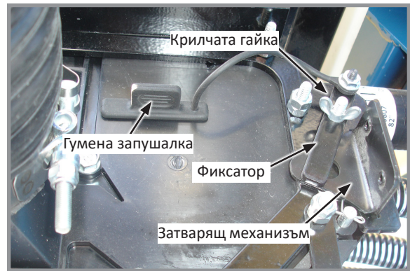
Механизъм за засмукване на система за зареждане на насипни материали (изглед отзад)
