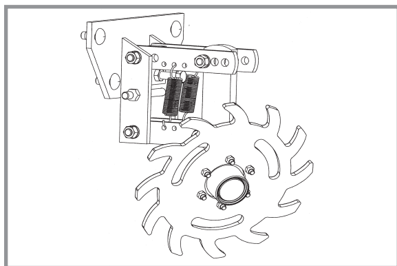
Монтирани на сееща секция колела за сътрнища
