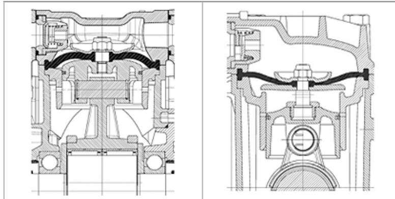
Полухидравлична помпа
