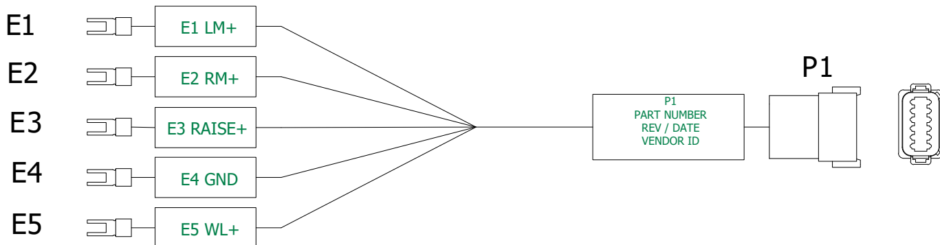
Схема за свързване на проводници, P/N 10172501
