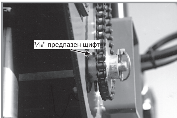
Трансмисионен вал
