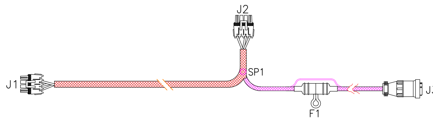
Схема за свързване на проводници, P/N A13944
