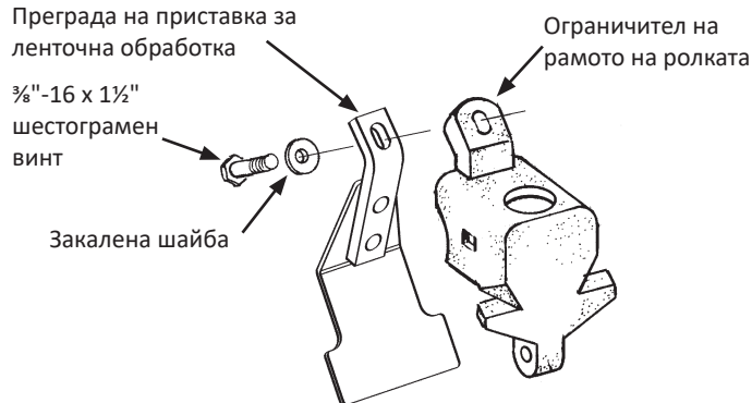
Монтиране на преграда на приставка за ленточна обработка с гранулирани химични препарати
