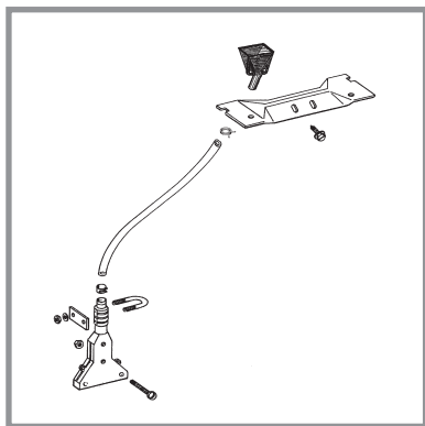
Приставка за 4½" (115 мм) ленточна обработка с компенсиране на наклона
