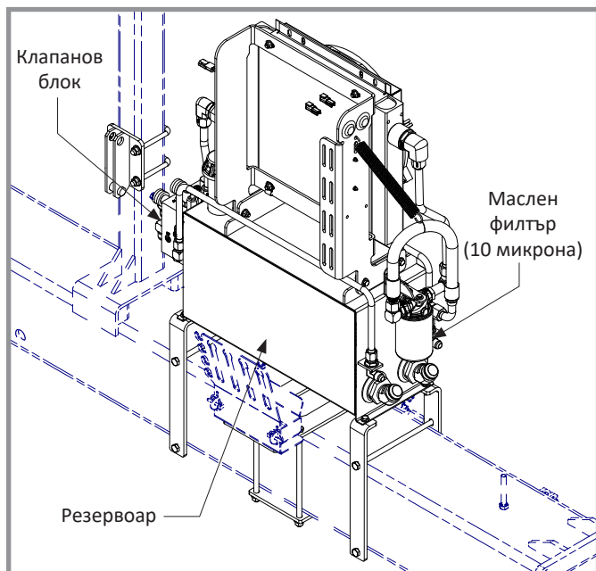
Двустепенен BOM -- Вакуум/Зареждане на насипни материали
