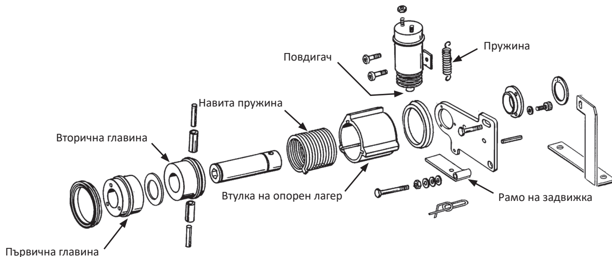
Основни части на еднокоростния съединител за редове
