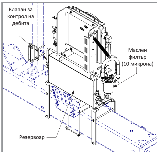
Едностепенен BOM -- Вакуум/Бункери на сееща секция
