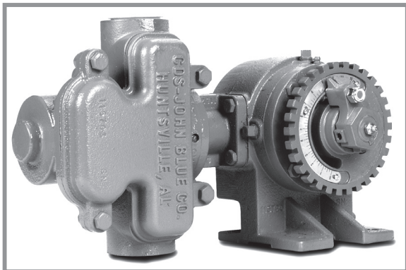
Бутална помпа
