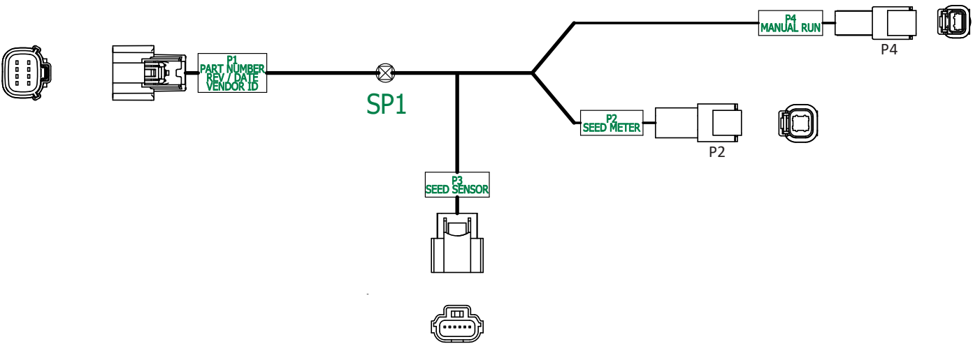
Схема за свързване на проводници, P/N A25038/A25039
