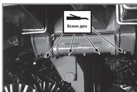
Панти на крило - 4 на крило
