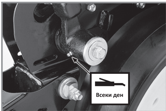
Рамена на габаритно колело - 1 на рамо (Уплътненията при рамото на габаритното колело се монтират с улея навън, за да може смазката да почисти замърсяванията от уплътнението. Изпомпвайте смазката към рамото до появата на нова смазка между шайбите и рамото.)
