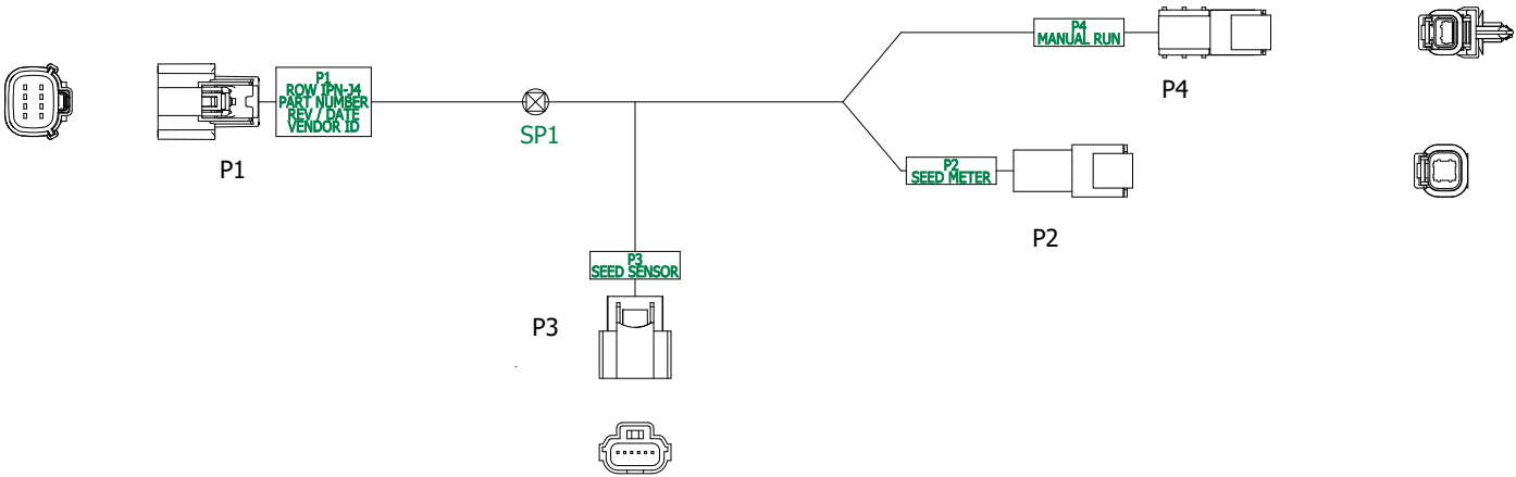
Схема за свързване на проводници, P/N A25203
