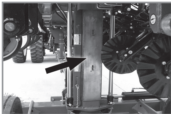
Централна стойка
