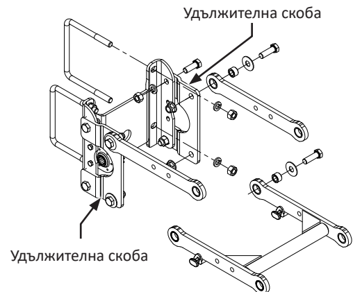
Удължителни скоби на сееща секция
