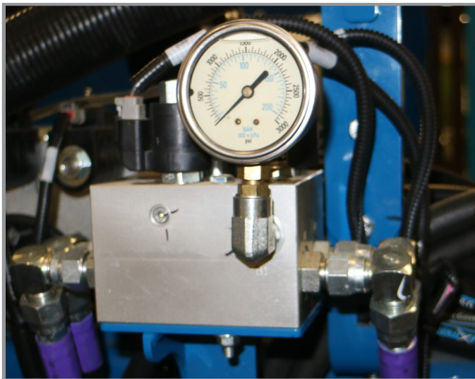
Манометр системы True Depth
