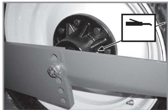
Подшипники транспортных колес — по 1 на ступицу
