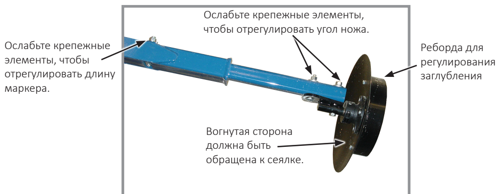
Регулировка угла дискового ножа маркера
