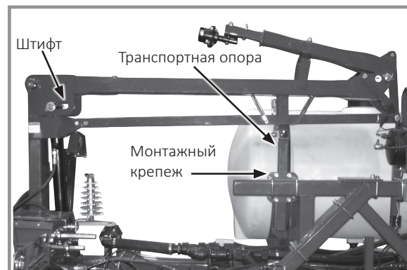
Транспортная опора маркера
