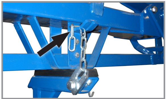
Стопорное устройство маркера
