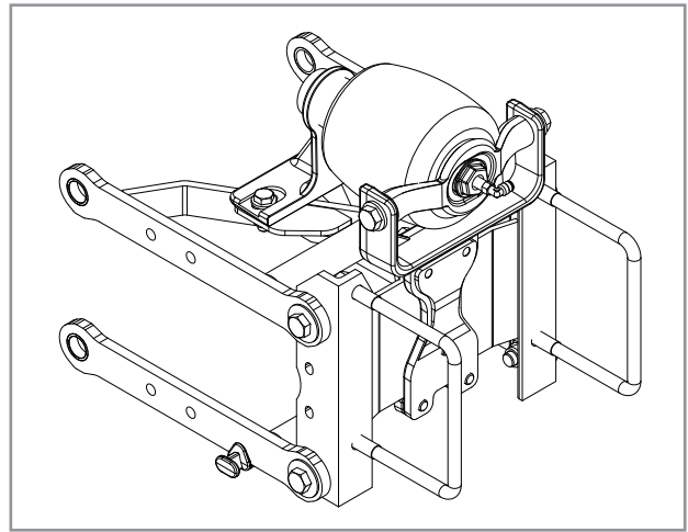
Пневмобалонна пружина фронтальної висівної секції
