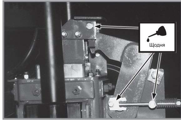
Запобіжний крук у верхній частині центральної секції
