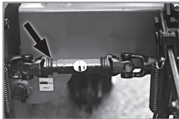
Ковзаючий елемент U-подібного з'єднання
