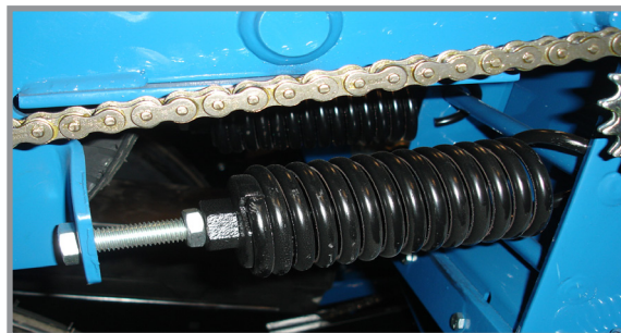
Пружини контактного привода
