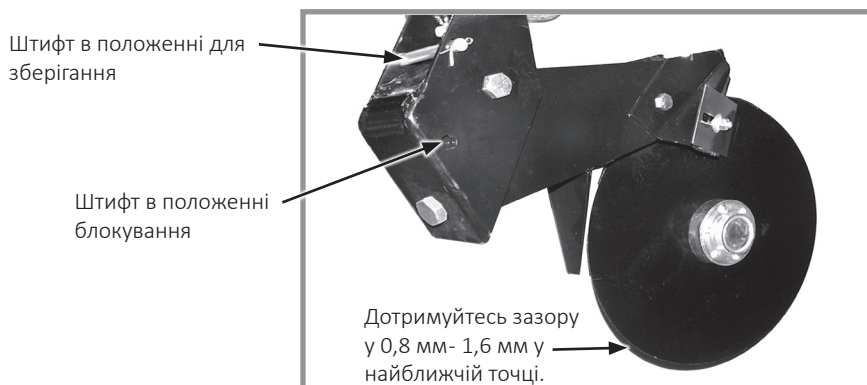
Дводисковий сошник для внесення добрив
