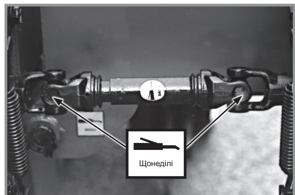
U-подібні з'єднання — по 2 на область шарнірного з'єднання
