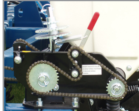
Привід трансмісії норми внесення добрив
