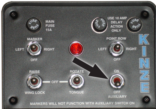
Допоміжний перемикач
