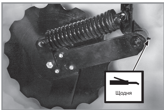
Зубчастий односторовий сошник для внесення добрив - 1
