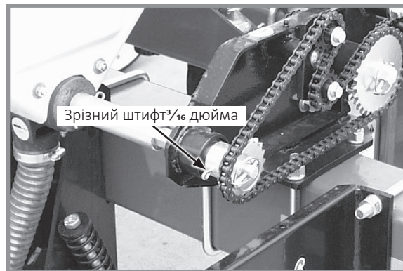
Трансмісія навісного обладнання для внесення сухих добрив
