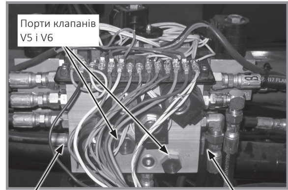
Гідравлічні порти A9 і B9
