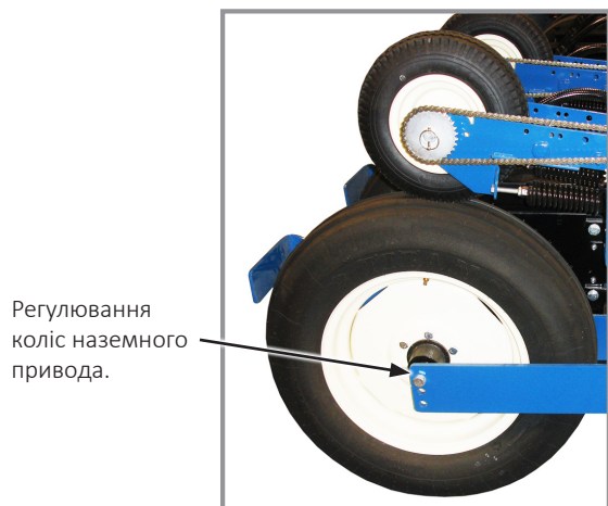
Регулювання коліс наземного привода
