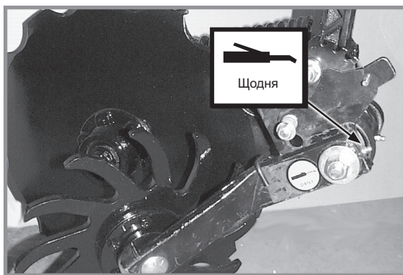
Обладнання у вигляді коліс для поживних залишків для використання з зубчастим односторовим сошником для внесення добрив
