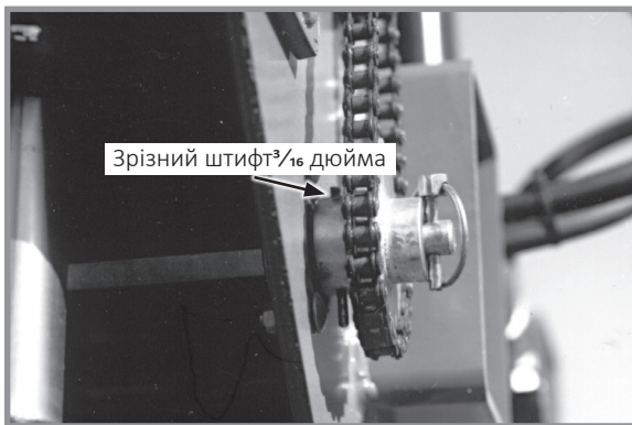
Вал трансмісії
