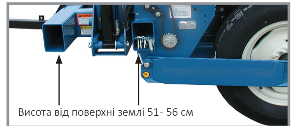
Вирівнювання рами сівалки
