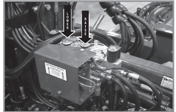
Регулювання органів управління швидкістю маркерів ряду
