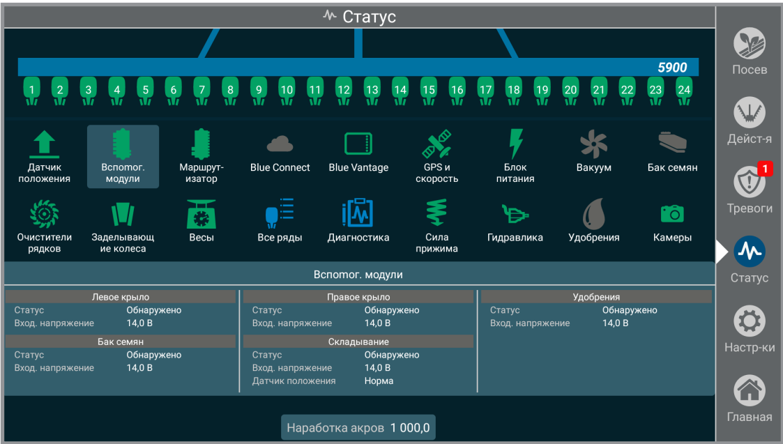
Использование вспомогательных модулей в зависимости от модели сеялки
