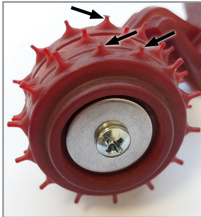
Виштовхуюче колесо з пошкодженими штифтами, позначені стрілками
