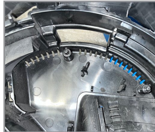
Сингулятор знято
