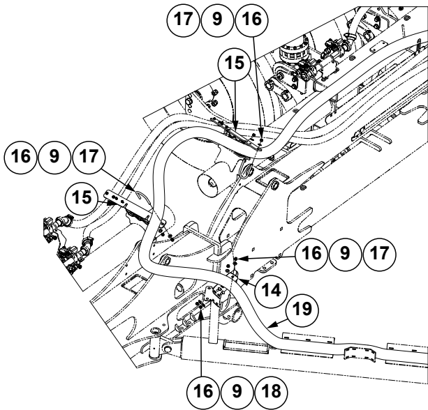
R.H. Draft Link Pivot - 24 Row
